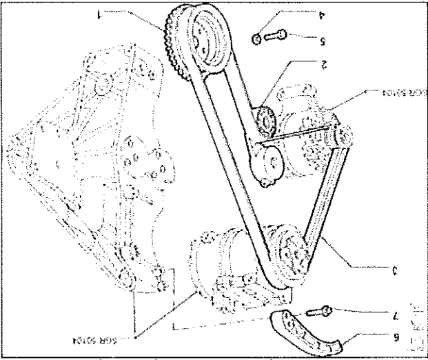
Slika 1 - Zatezač ili španer klinastog kaiša pod rb.2
